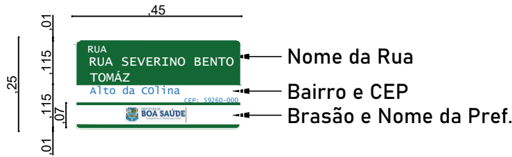
DETALHE CALÇADA Sem Escala
