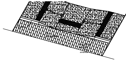
PERSPECTIVA REBAIXAMENTO DE CALÇADA (RAMPA) Sem Escala
