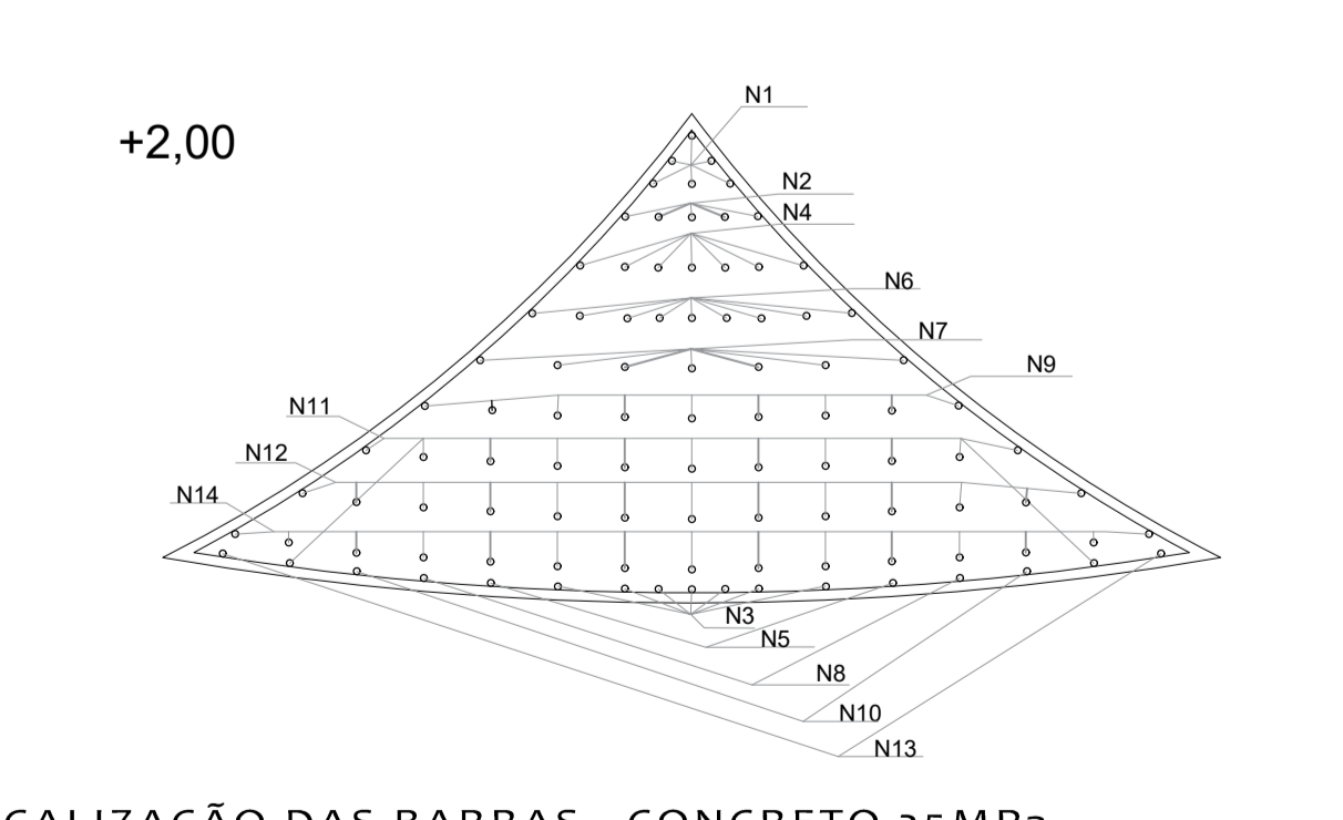
LOCALIZAÇÃO DAS BARRAS - CONCRETO 25MPa Escala _____ 1/50
